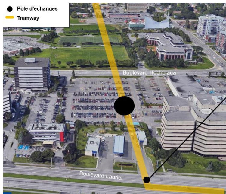
Figure 13 Insertion du tramway dans l'axe Roland-Beaudin au sud du boulevard Hochelaga, scénario modifié retenu
