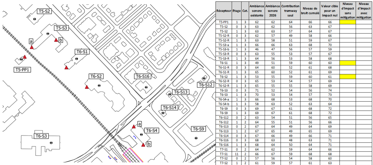
Figure 16 : Niveaux sonores et niveaux d'impact correspondants après mise en place des mesures de réduction à la source – Secteur pôle Sainte-Foy – Partie 1 - Échelle1/3000e
