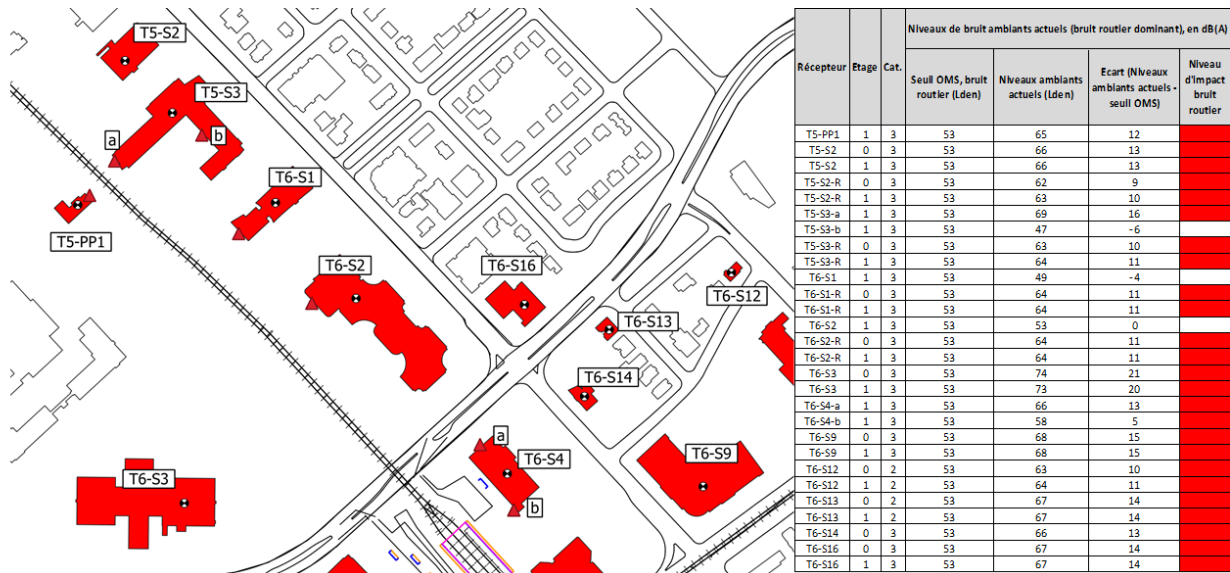
Figure 19 : Niveaux sonores et niveaux d'impact du bruits ambiants actuels (bruit routier dominants) par rapport aux recommandations de l'OMS – Secteur Pôle Sainte-Foy – Partie 1 - Niveau de bruit L_{DEN} – Échelle 1/3000°
