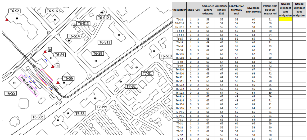
Figure 17 : Niveaux sonores et niveaux d'impact correspondants après mise en place des mesures de réduction à la source – Secteur pôle Sainte-Foy – Partie 2 - Échelle1/3000e
