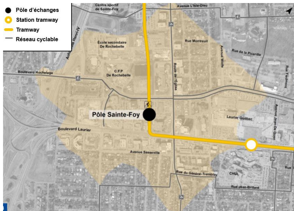
Figure 16 Desserte du pôle d'échanges de Sainte-Foy (scénario modifié)
